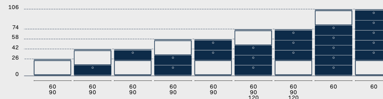
Larghezze moduli profondità 50,4 cm Widths for 50,4cm-deep units
